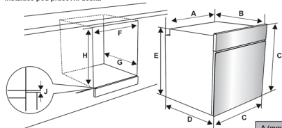
Instalace pod pracovní desku
