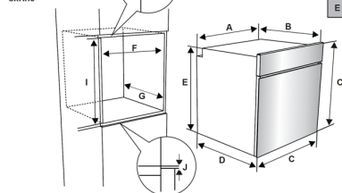
Instalace do nástěnné skříně
